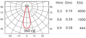
OSLON 1pcs(700mA) WW 36°
