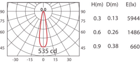
OSLON 1pcs(700mA) WW 24°
