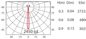
OSLON 1pcs(700mA) WW 8°
