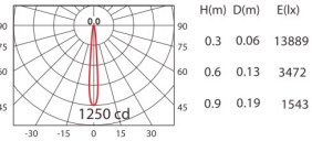
OSLON 1pcs(700mA) WW 12°
