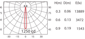
OSLON 1pcs(700mA) WW 12°
