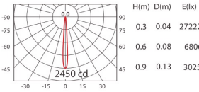
OSLON 1pcs(700mA) WW 8°
