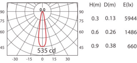
OSLON 1pcs(700mA) WW 24°
