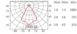
CoB 4700lm 1050mA WW 70°
